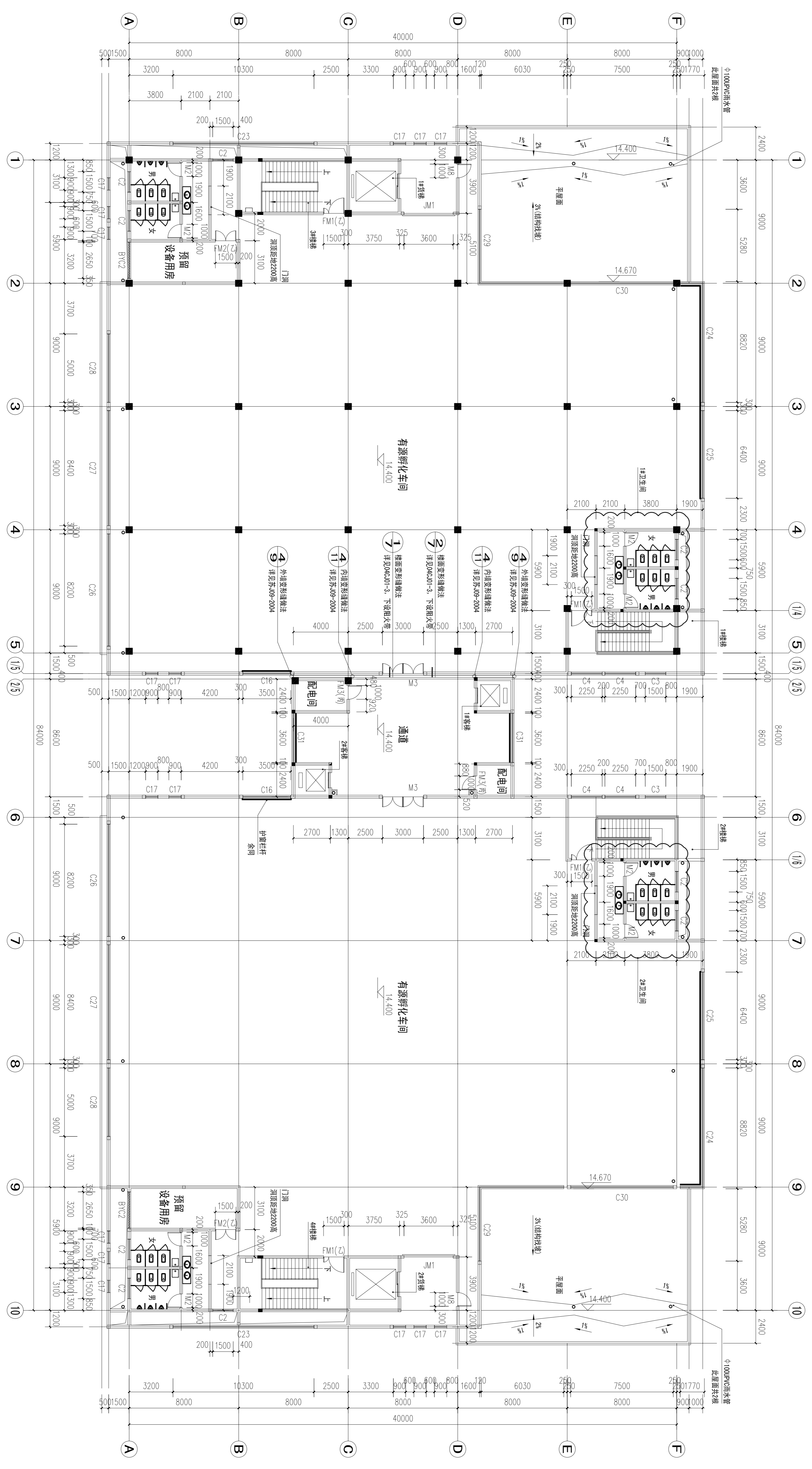
四层平面图 1:150 (本层建筑面积为3175M 2 )
